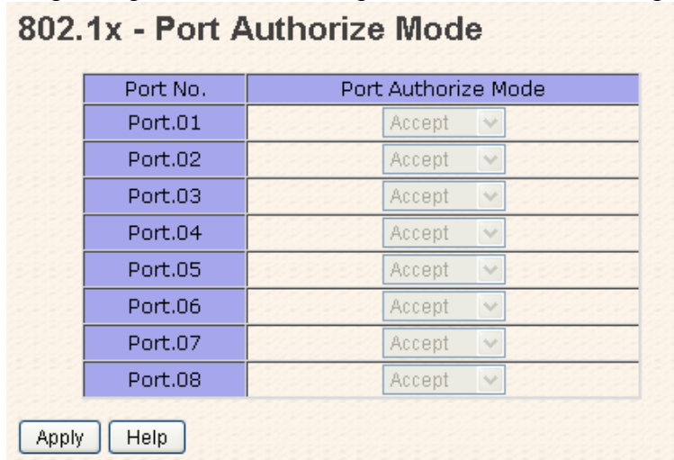
Рис. Интерфейс 802.1x - Режим авторизации по портам
