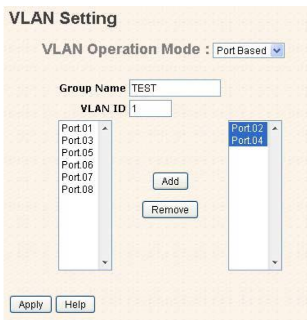
Рис.2. Настройка VLAN на основе портов
