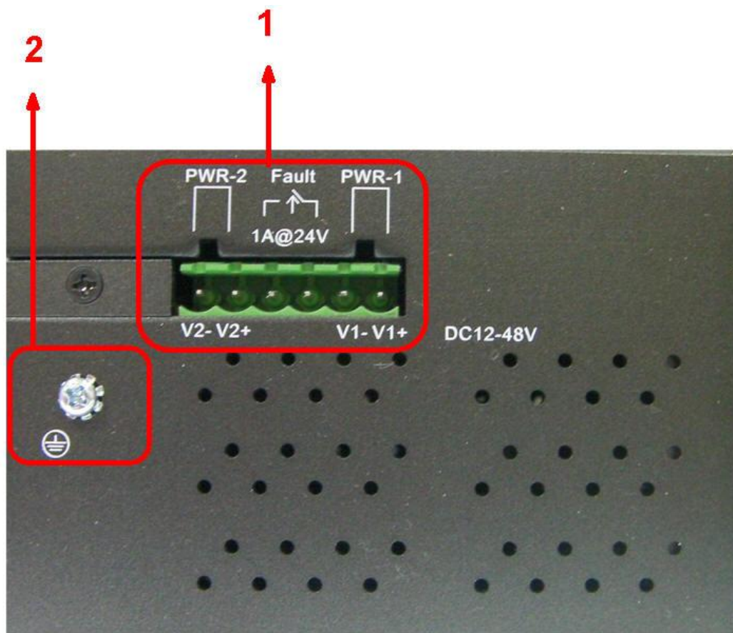
Рис. Подключение питания к SWMG-44(SFP)GC-W
